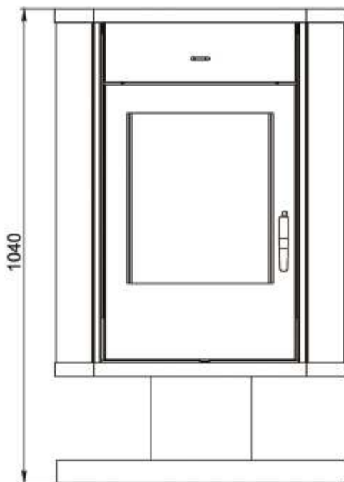
Вид спереди
