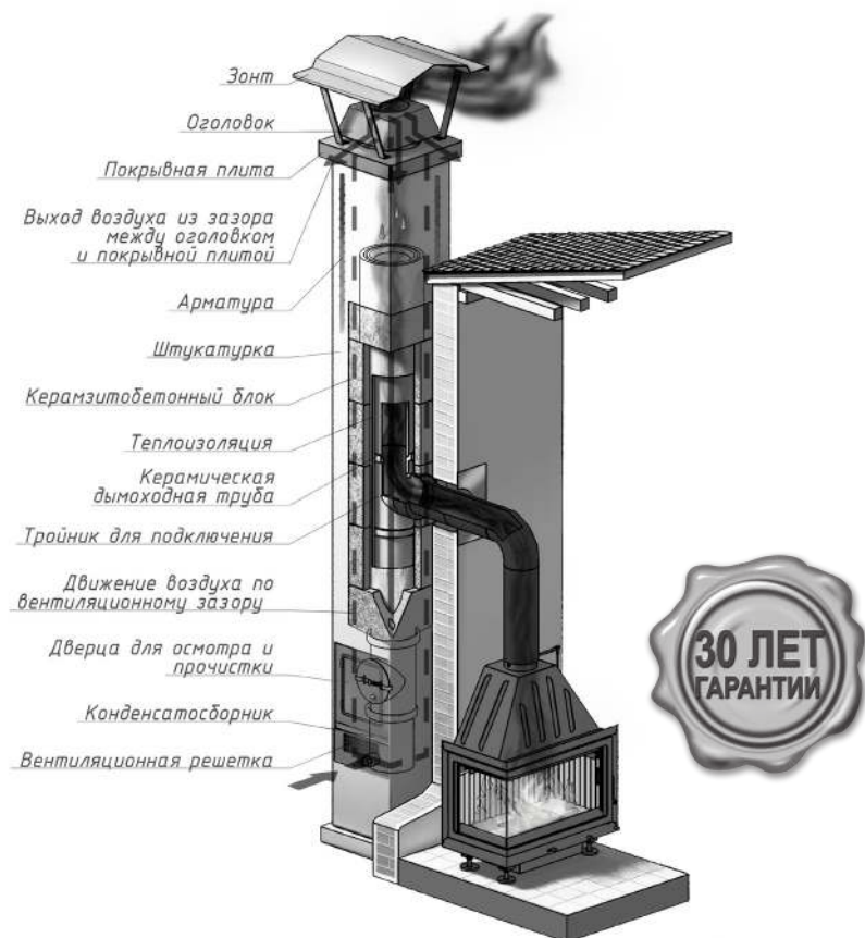
Движения потоков в дымоходной системе Ecosmose
